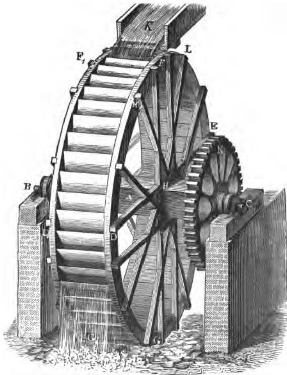
Fig. 14. Oberschlächtiges Wasserrad.
